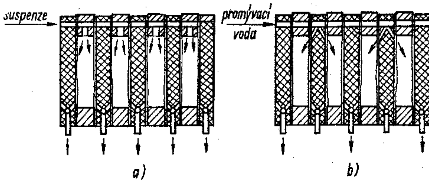
Obr. 2 Kalolis (tlakový filtr) - princip činnosti
