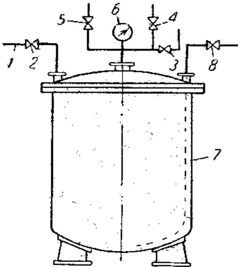
Obr. 25 Schéma monžiku
