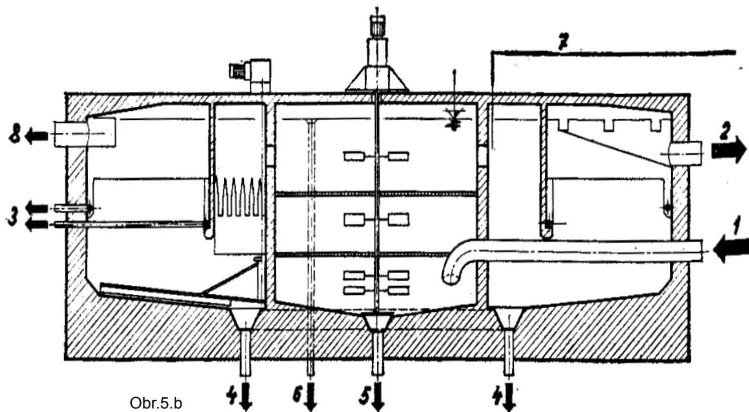
Obr. 99. Čiřič Binar-Bělský modifikovaný pro použití pomocných flokulantů
