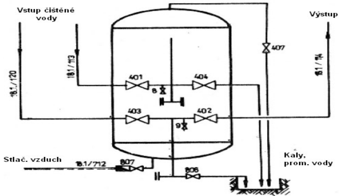
Obr. 1 Pískový filtr
